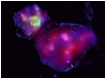
DEM L316 (Chandra/NOAO)
